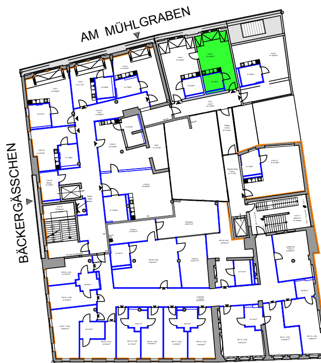
ÜBERSICHTSGRUNDRISS
