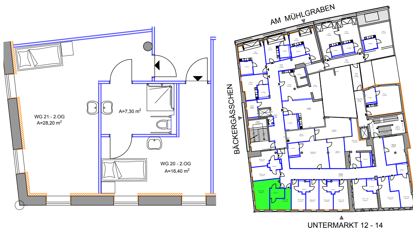
ÜBERSICHTSGRUNDRISS
